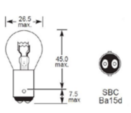
BA15D (level pins)
